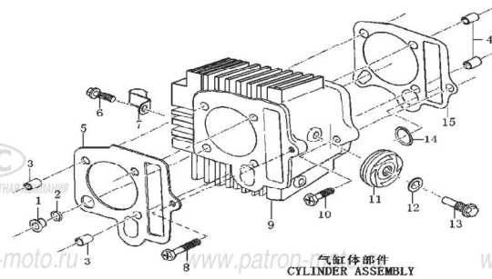
Рис. 2 ЦИЛИНДР В СБ.
