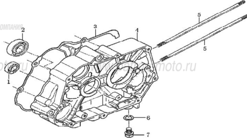
Рис. 9 ПОЛУКАРТЕР ПРАВЫЙ
