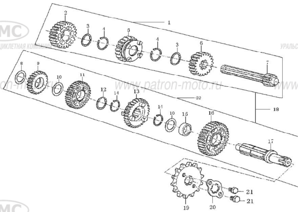
Рис. 11 КОРОБКА ПЕРЕДАЧ
