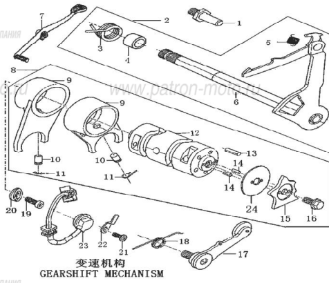
Рис. 13 МЕХАНИЗМ ПЕРЕКЛЮЧЕНИЯ ПЕРЕДАЧ
