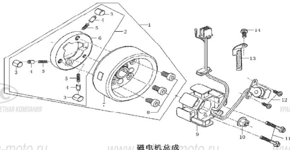
Рис. 14 МАГНЕТО В СБ.
