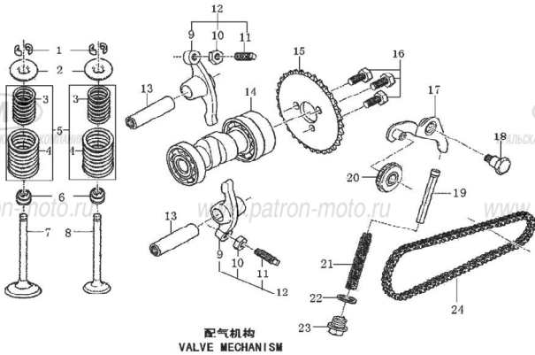
Рис. 3 МЕХАНИЗМ ГАЗОРАЗРЕДЕЛЕНИЯ
