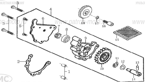
Рис. 7 МАСЛОНАСОС В СБ.
