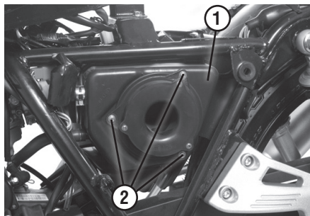
Рис. 17. Воздухофильтр
