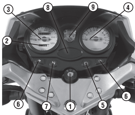
Рис. 7. Панель приборов
