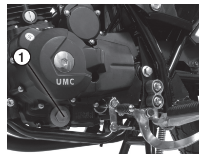
Рис. 12. Крышка масляного фильтра и пробка сливного отверстия
