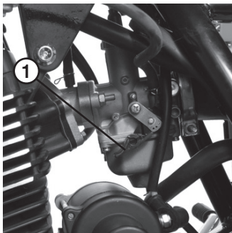
Рис. 9. Рычажок топливного корректора
