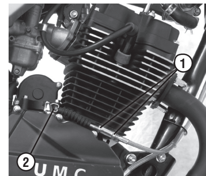
Рис. 13. Регулировка сцепления
