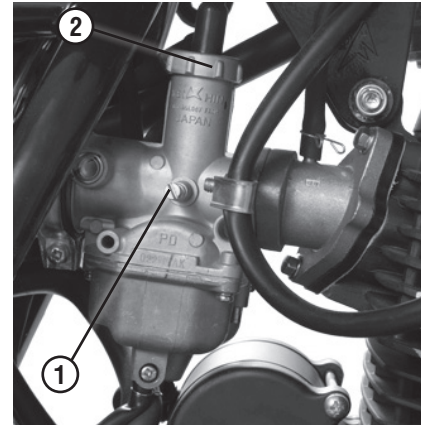
Рис. 18. Карбюратор
