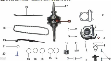
Рис. 29 Цилиндр в сб., Вал коленчатый в сб., Поршень в сб.
