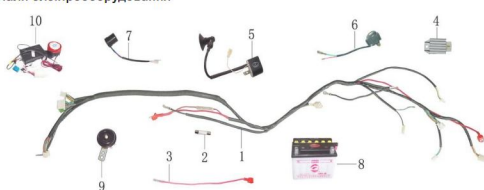
Рис. 19 Детали электрооборудования
