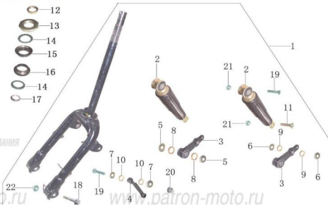
Рис. 5 Вилка передняя в сб.
