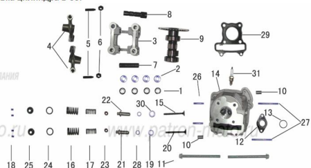
Рис. 28 Головка цилиндра в сб.
