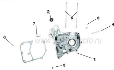
Рис. 37 Полукартер правый в сб.
