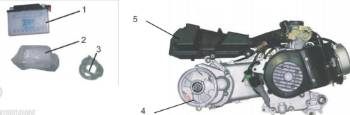
Рис. 5 Двигатель в сб., Аккумулятор
