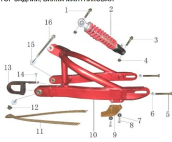
Рис. 16 АМОРТИЗАТОР ЗАДНИЙ, ВИЛКА МАЯТНИКОВАЯ
