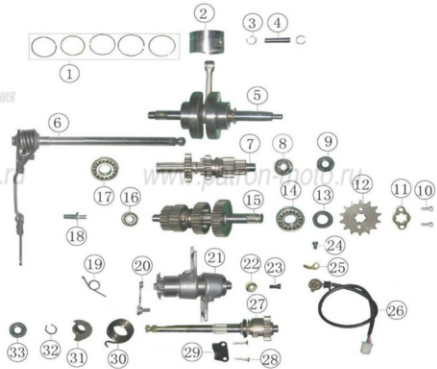
Рис. 3 ПОРШНЕВАЯ ГРУППА, СИСТЕМА ТРАНСМИССИИ, СИСТЕМА ПЕРЕКЛЮЧЕНИЯ ПЕРЕДАЧ
