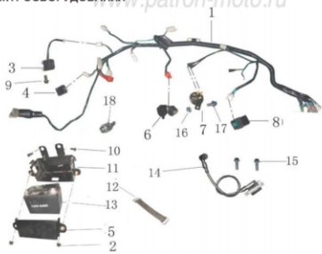
Рис. 15 ДЕТАЛИ ЭЛЕКТРООБОРУДОВАНИЯ
