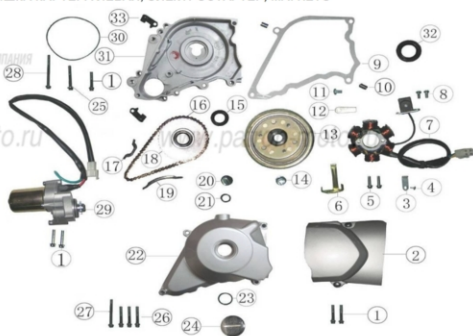
Рис. 6 КРЫШКА КАРТЕРА ЛЕВАЯ, ЭЛЕКТРОСТАРТЕР, МАГНЕТО
