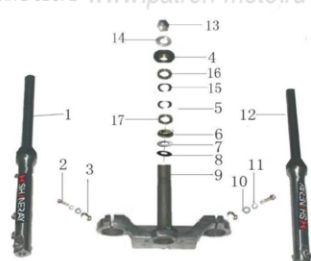
Рис. 9 ВИЛКА ПЕРЕДНЯЯ В СБОРЕ
