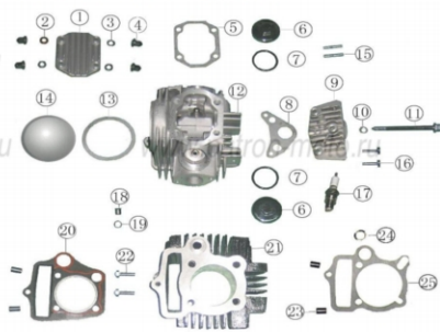
Рис. 1 ГОЛОВКА ЦИЛИНДРА В СБОРЕ, ЦИЛИНДР В СБОРЕ
