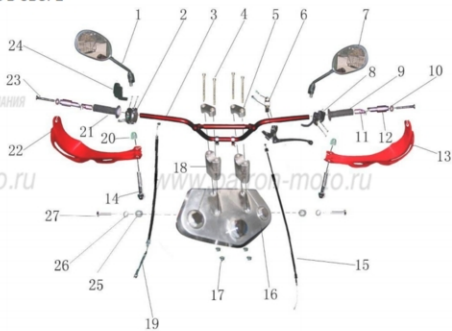
Рис. 8 РУЛЬ В СБОРЕ
