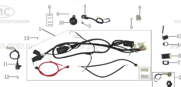
Рис. 12 ДЕТАЛИ ЭЛЕКТРООБОРУДОВАНИЯ
