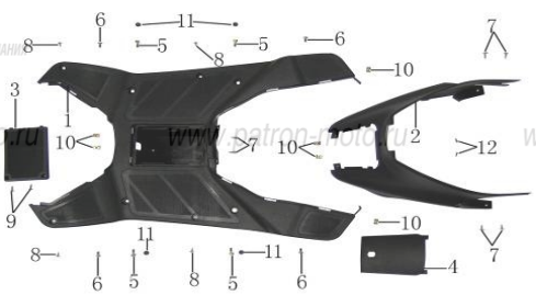
Рис. 7 ОБЛИЦОВКА ПОЛА В СБОРЕ
