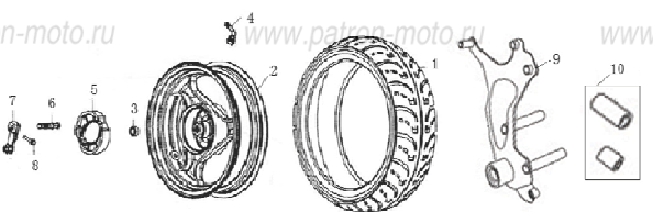
Рис. 12 Колесо заднее в сб.
