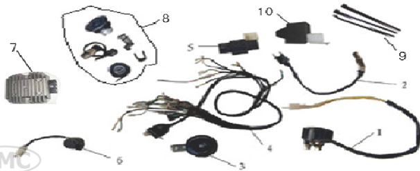
Рис. 10 Детали электрооборудования
