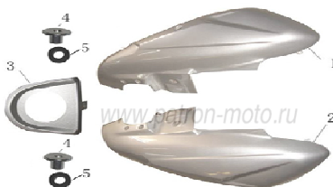
Рис. 6 Обтекатель седла
