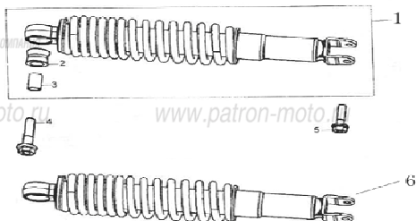
Рис. 17 Амортизатор задний
