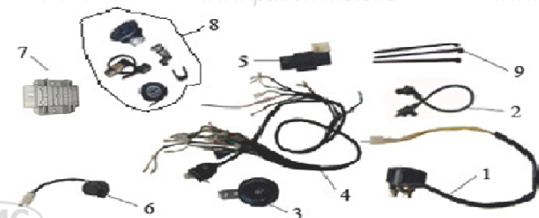
Рис. 10 Детали электрооборудования
