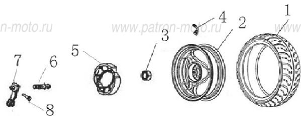
Рис. 12 Колесо заднее в сб.
