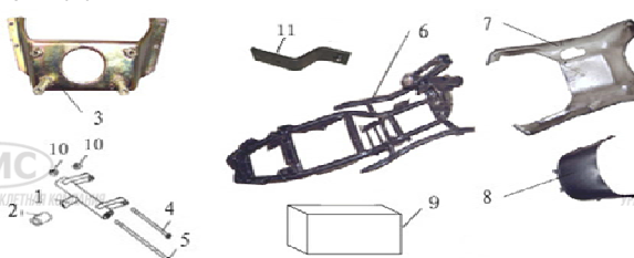
Рис. 21 Рама
