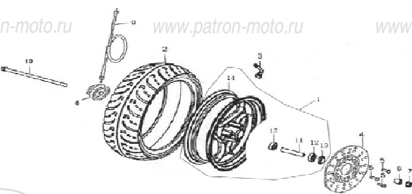
Рис. 11 Колесо переднее в сб.
