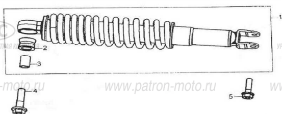
Рис. 17 Амортизатор задний
