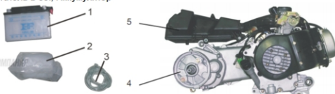
Рис. 4 Двигатель в сб., Аккумулятор
